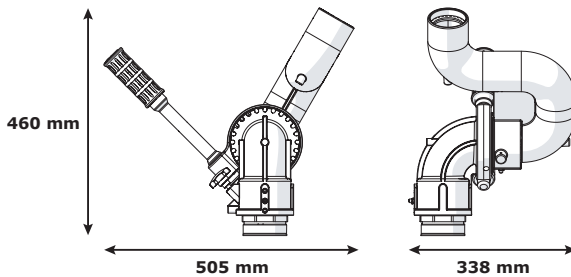
Ρύθμιση οριζόντιας κίνησης με κοχλία. Υποδοχή λίπανσης.
